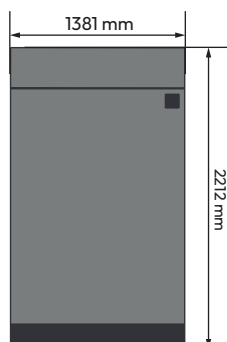
Boční pohled
