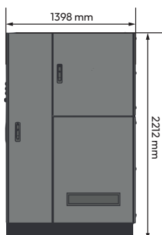
Boční pohled
